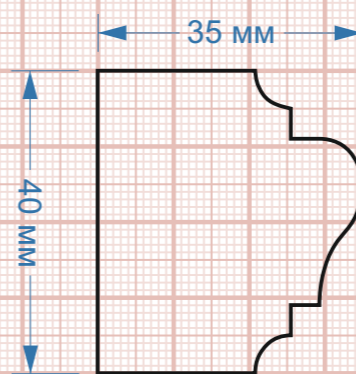
Молдинг иМ-2 40Нх35 мм
