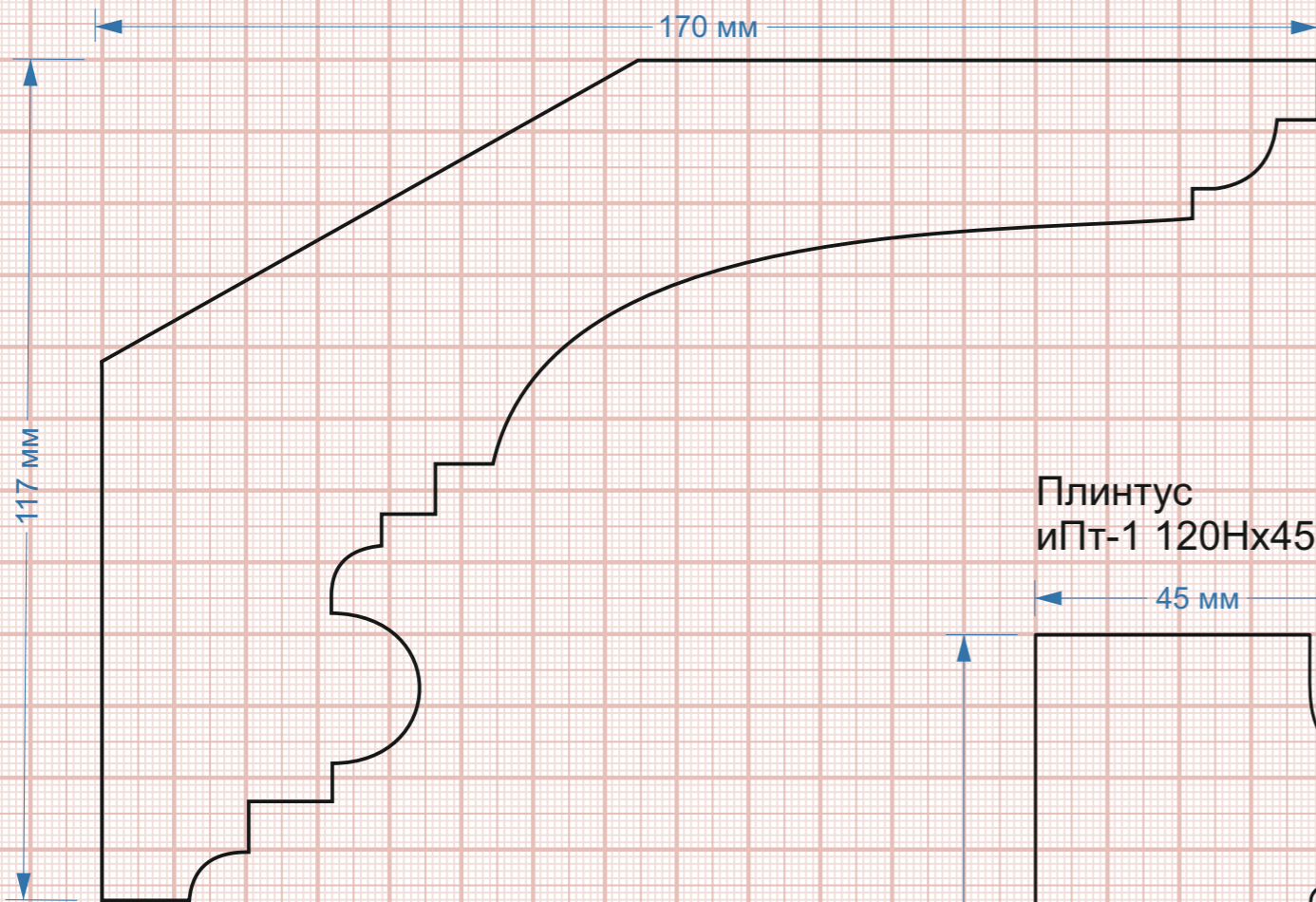
Карниз иКТ-1 117Нх170 мм
