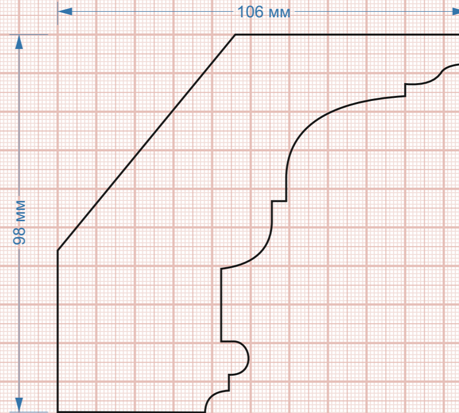
Карниз иКТ-4 98Нх106 мм
