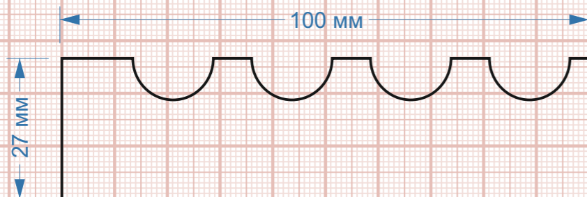
Молдинг иМ-6 100Нх27 мм
