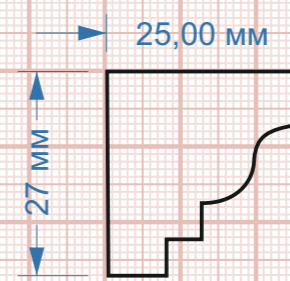
Молдинг иМ-3 27Нх25 мм
