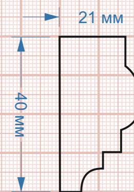
Молдинг иМ-5 40Нх21 мм
