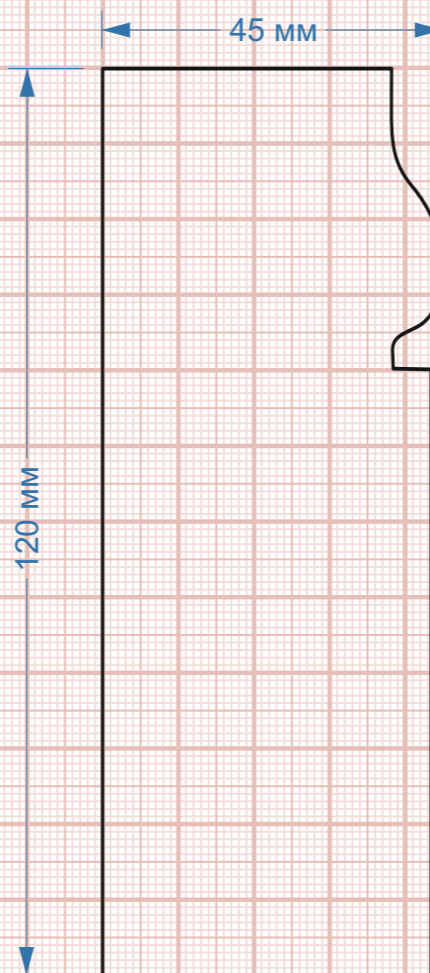
Плинтус иПТ-1 120Нх45 мм
